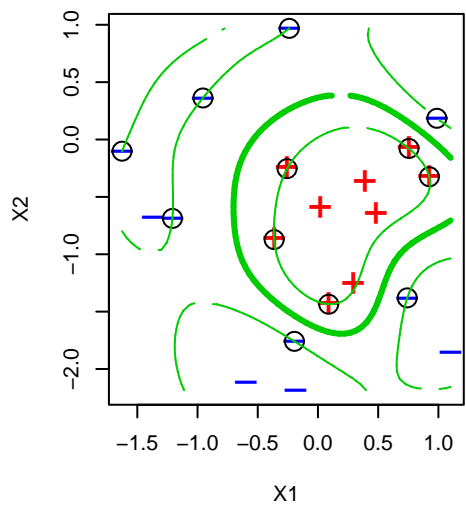
lambda= 0.216
